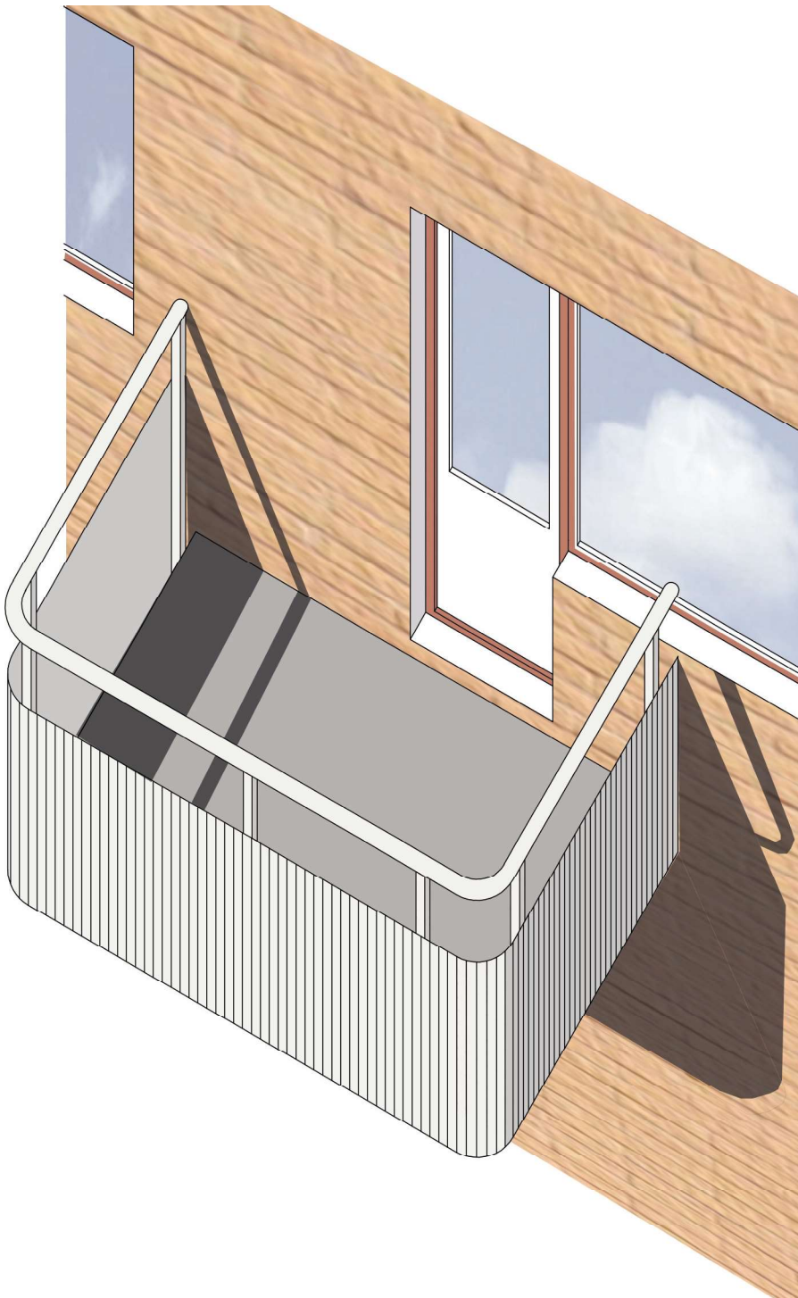
Isometriskt perspektiv Balkongräcke typ 1
