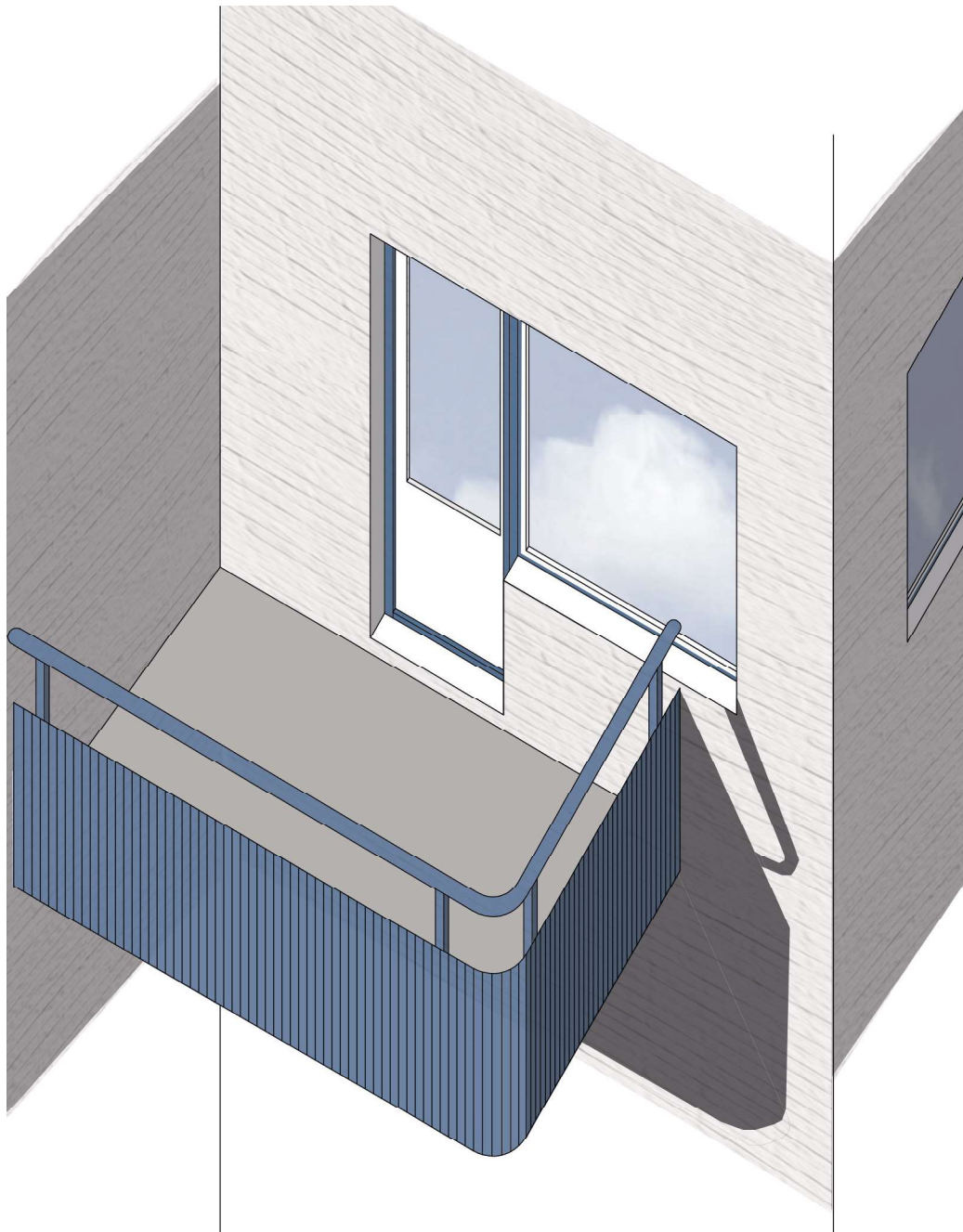
Isometriskt perspektiv Balkongräcke typ 2
